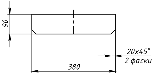
Поз.2 (Ребро)
