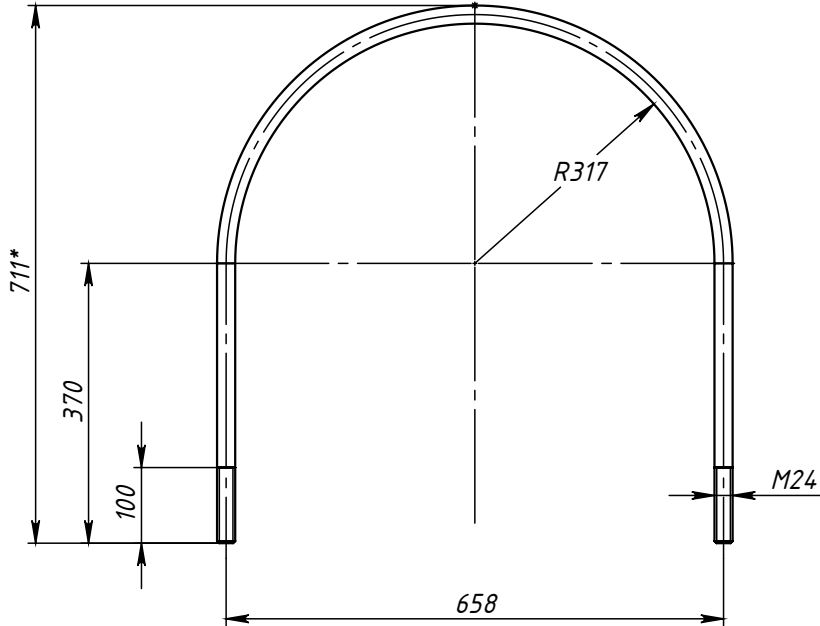
Поз.6 (Упор)
