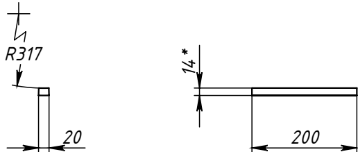
Поз.6 (Упор)
